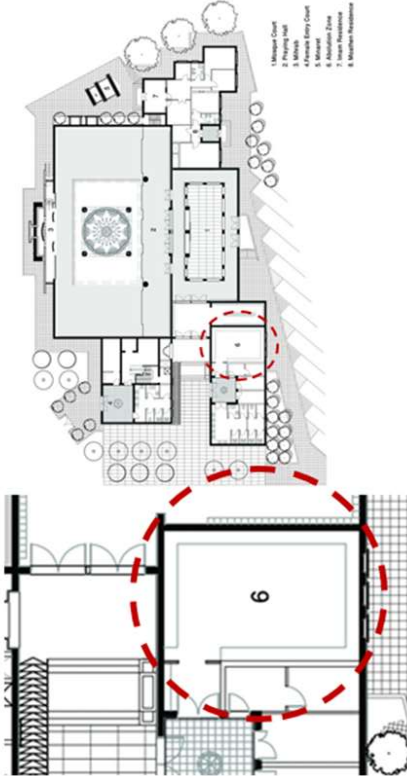
شكل " ٣٠ " المسقط الأفقي لإحدى المساجد لوضع رؤية تصميمية معاصرة لمكان الوضوء تلي المتطلبات الضرورية للمتوضئ وتحد من الأضرار بالبيئة
