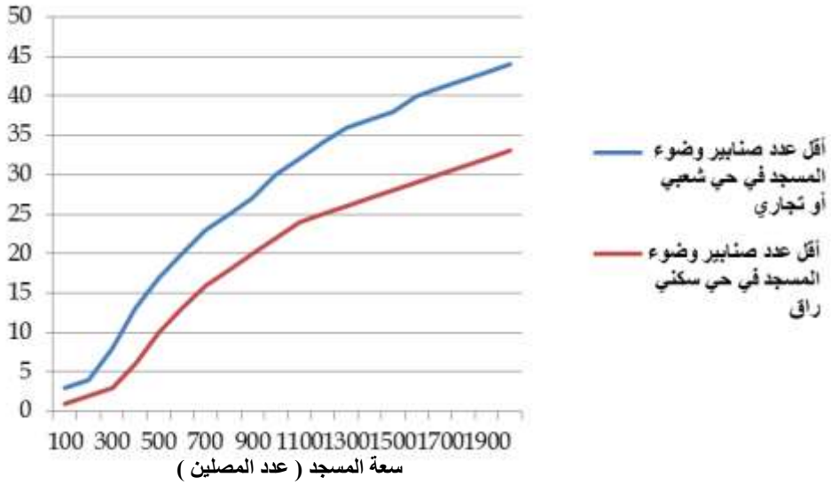
شكل " 15 " رسم بياني يوضح عدد صنابير الضوء المطلوبة للمسجد وفقا لمساحته
